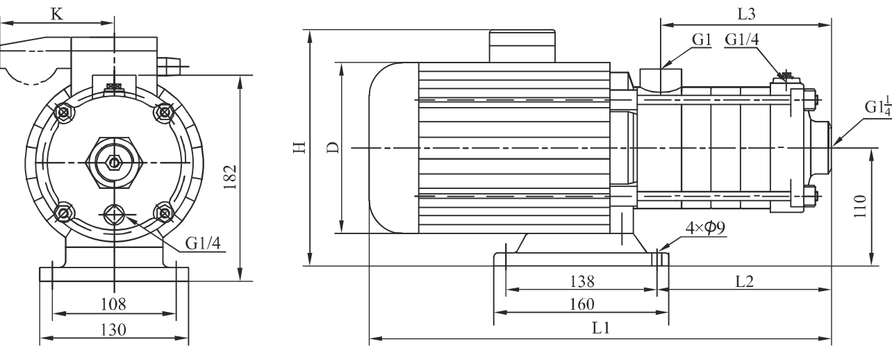
尺寸和重量
