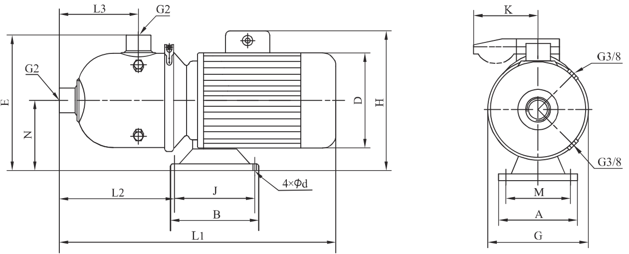
安装图
