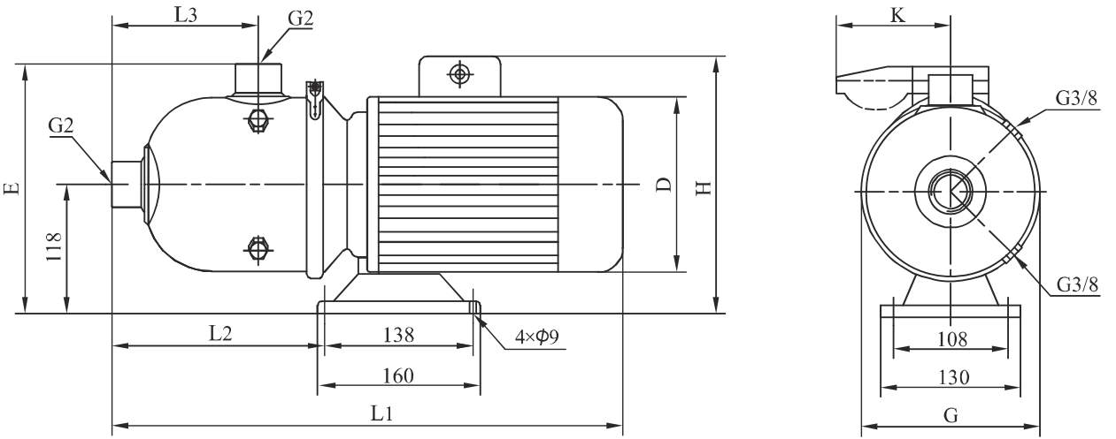
安装图
