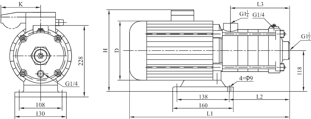
尺寸和重量
