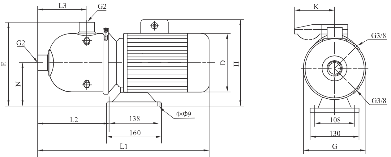
安装图
