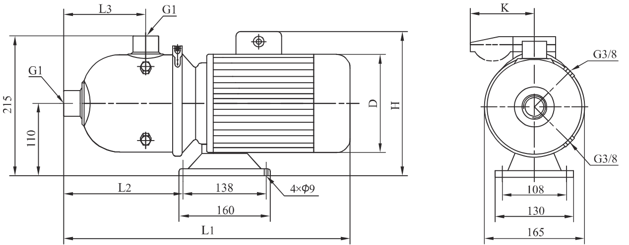
安装图
