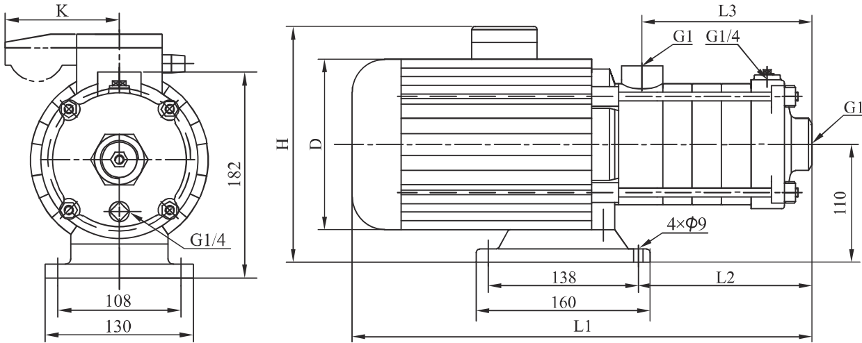
尺寸和重量
