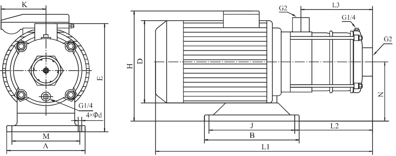
尺寸和重量
