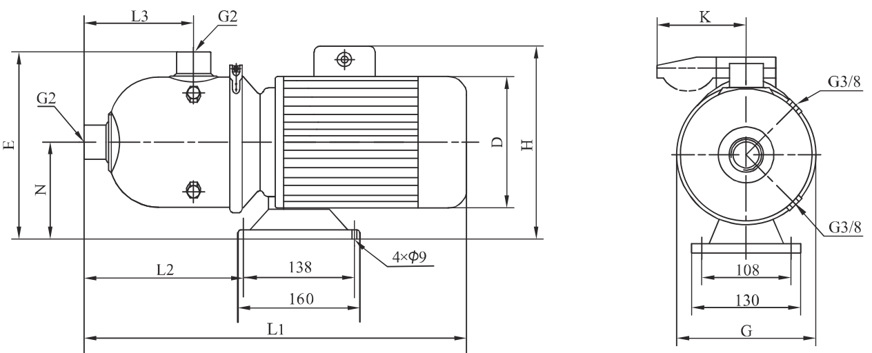
安装图
