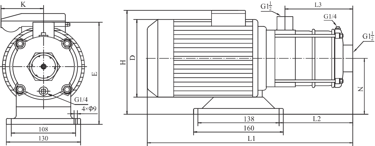
尺寸和重量
